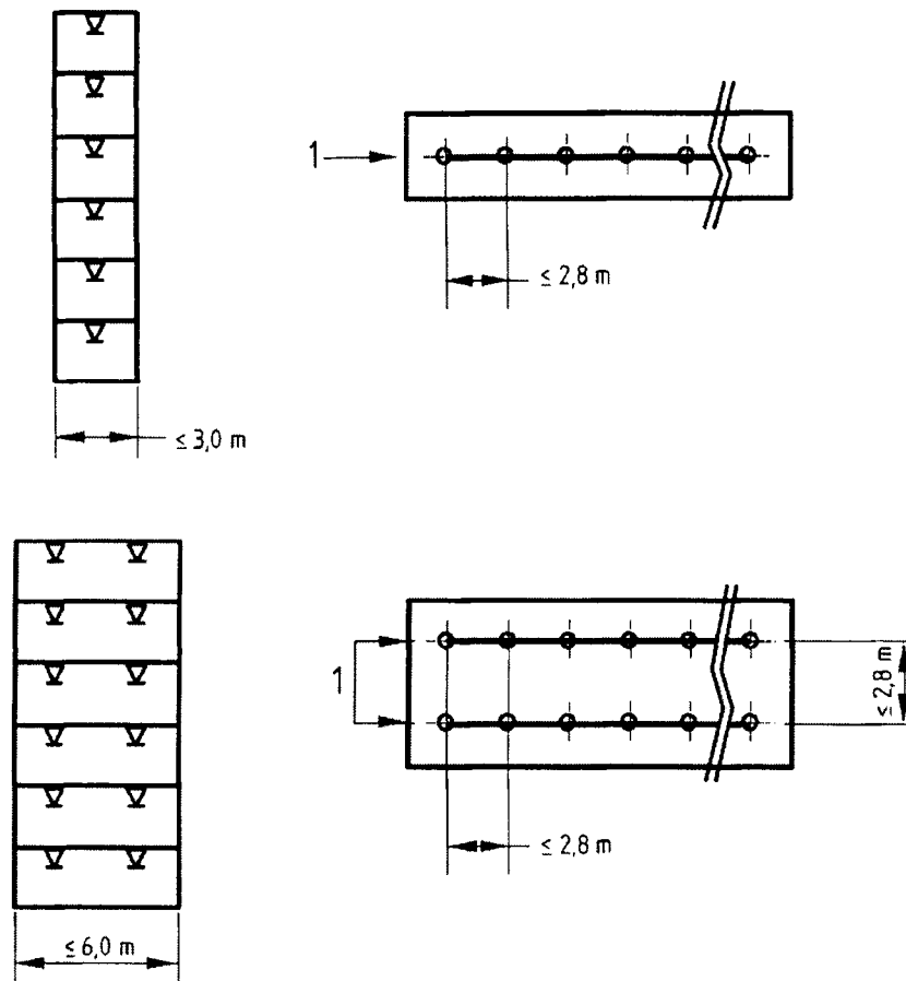
Рисунок 15 – Розміщення проміжних спринклерів у складських приміщеннях типу ST5 і ST6
