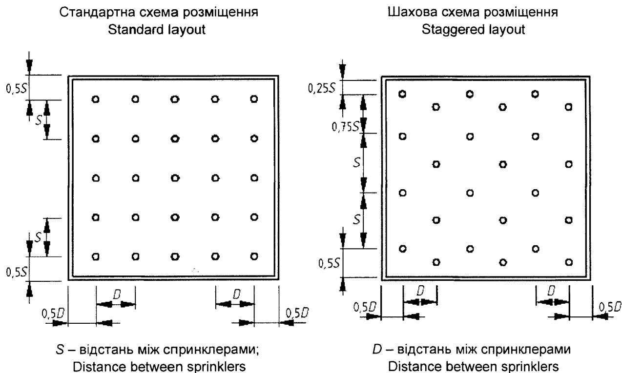
Рисунок 8 – Розміщення стельових спринклерів
