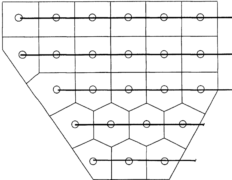
Рисунок 22 – Визначення площі, яку покриває один спринклер Figure 22 – Determination of area covered per sprinkler
