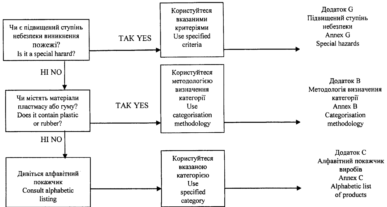
Рисунок 2 – Блок-схема для визначення класу складського приміщення за рівнем пожежної небезпеки
